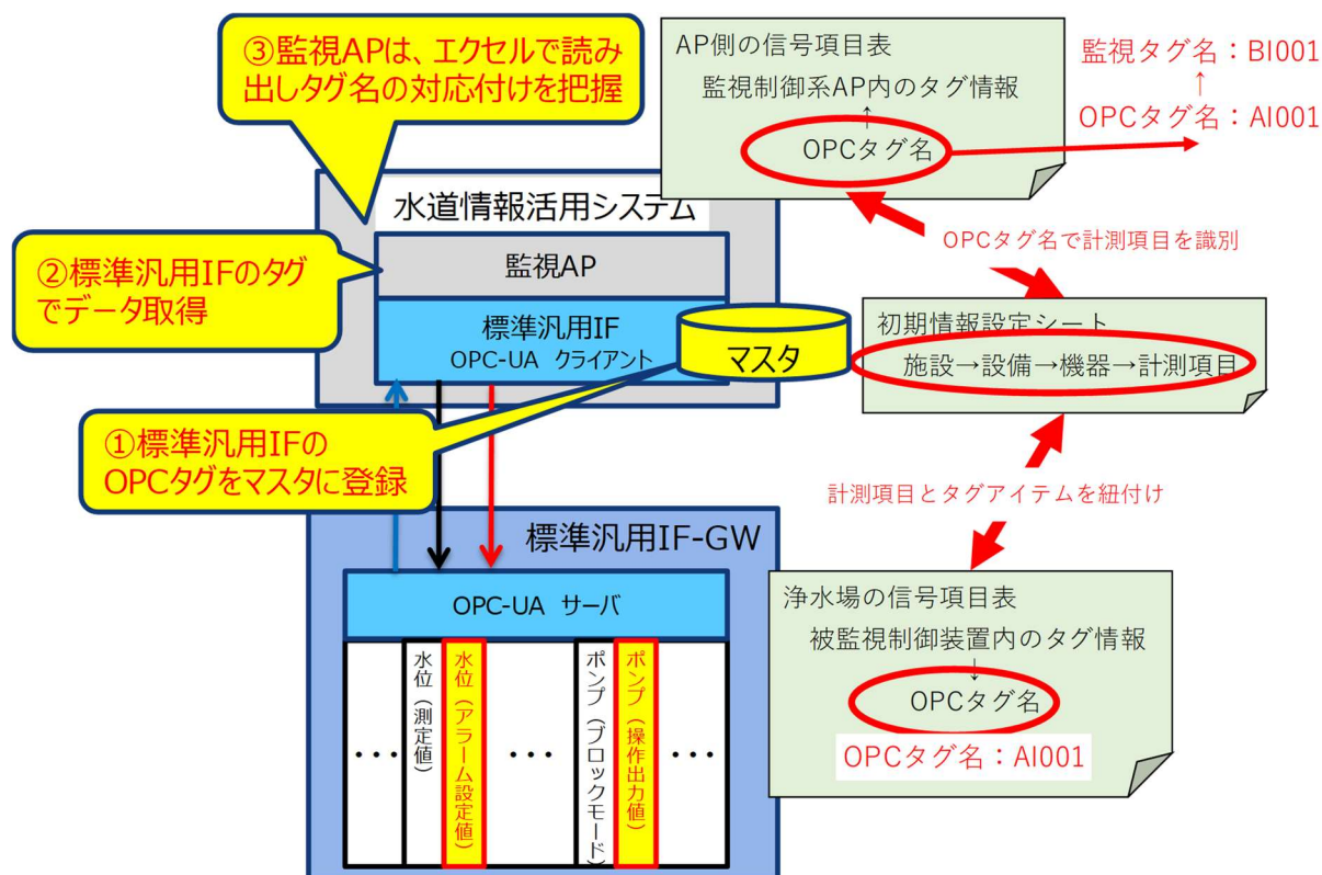
図 5-2 OPC タグ名を使った標準汎用 IF-GW と監視 AP とが連携する仕組み
