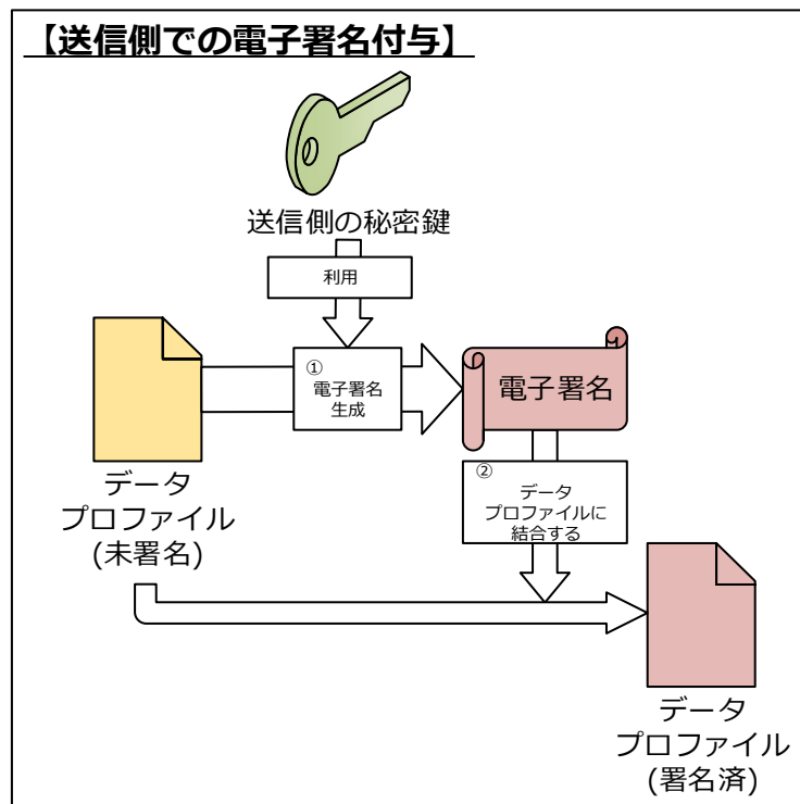
図 5-6:送信側での電子署名付与方式
